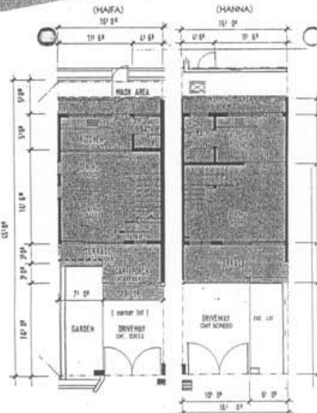
Pelan Tingkat Bawah Ground Floor Plan
